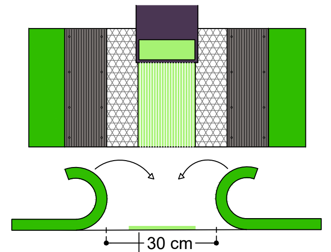
DETALL ENCOLAT JUNTES
