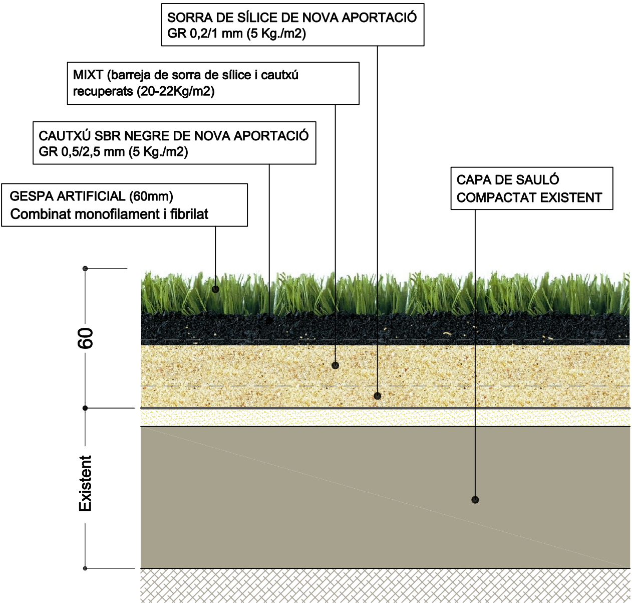
PERFIL CONSTRUCTIU CAMP DE FUTBOL 11 MUNICIPAL REDDIS
