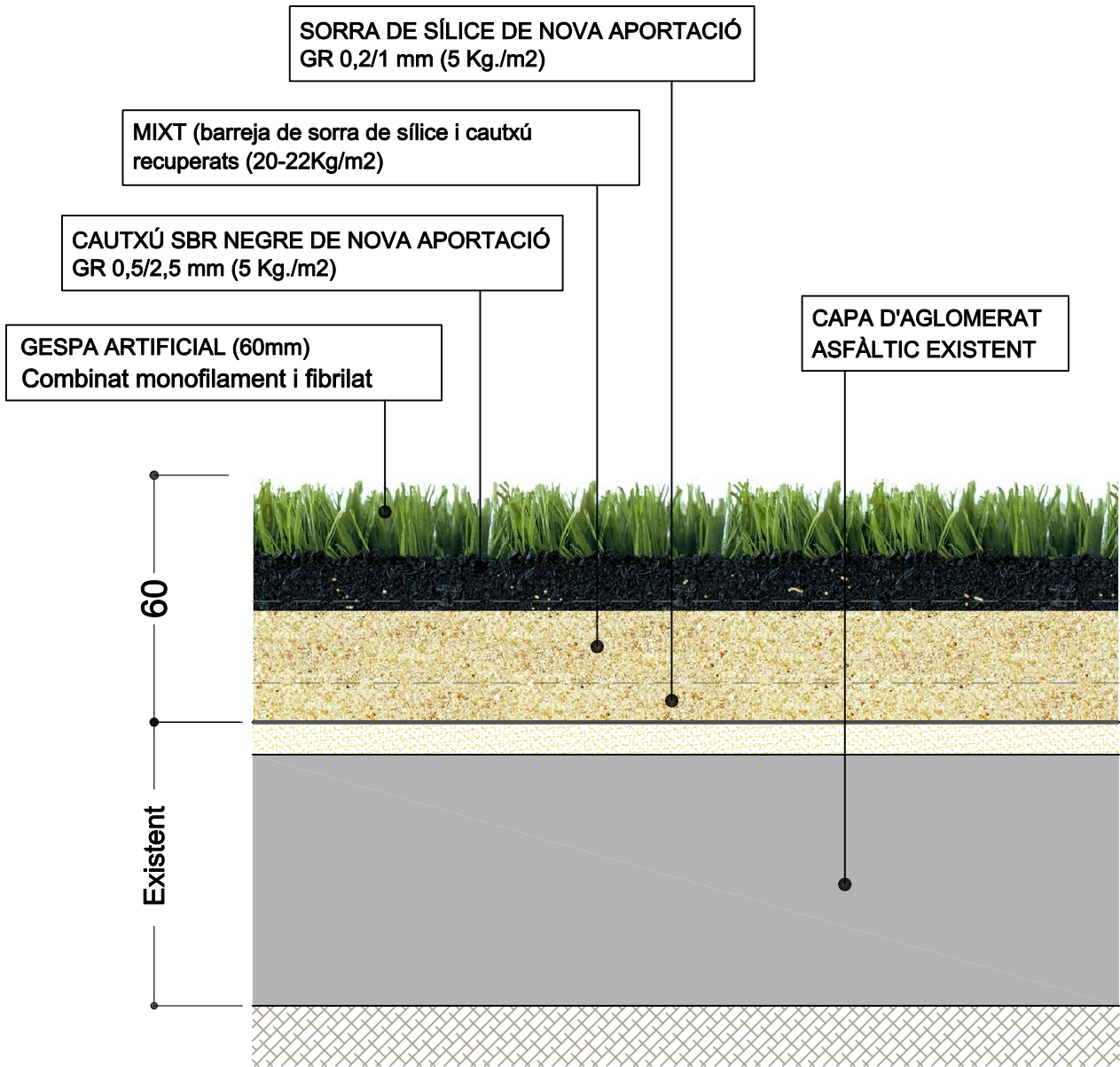
PERFIL CONSTRUCTIU CAMPS DE FUTBOL 11 LA PASTORETA I ANNEX ESTADI
