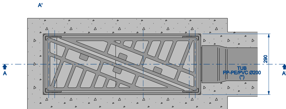
SECCIÓ A-A'
