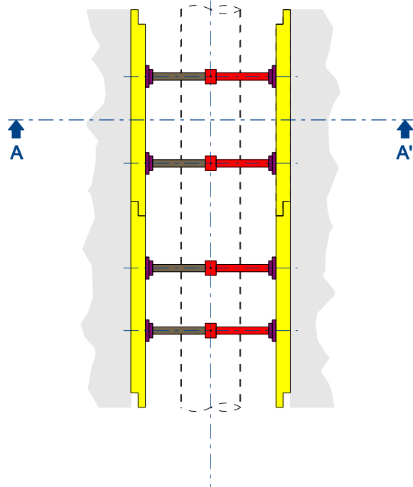
PLANTA
