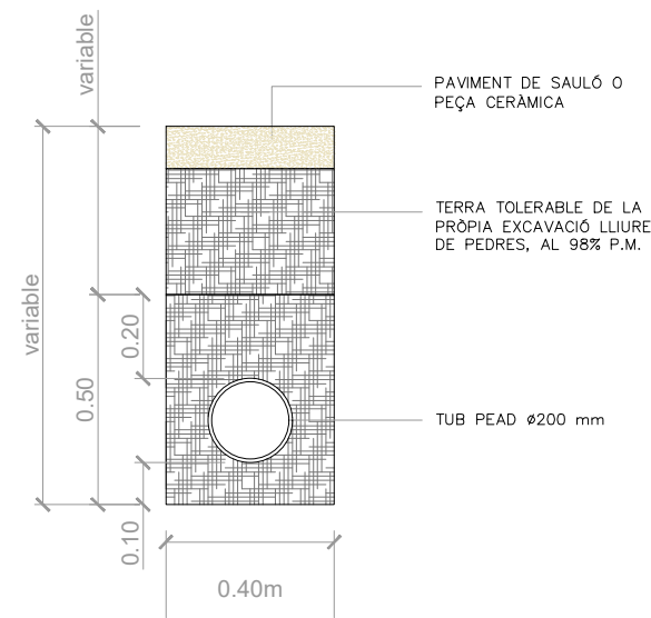
RP. DETALL RASA SOTA PAVIMENT
