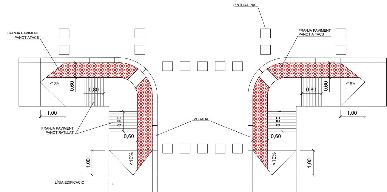
CREUAMENT A DIFERENT NIVELL AMB APLICACIÓ TÀCTIL EN LES CANTONADES ON ES BAIXA LA VORERA A NIVELL DE LA CALÇADA AMB VORADA
