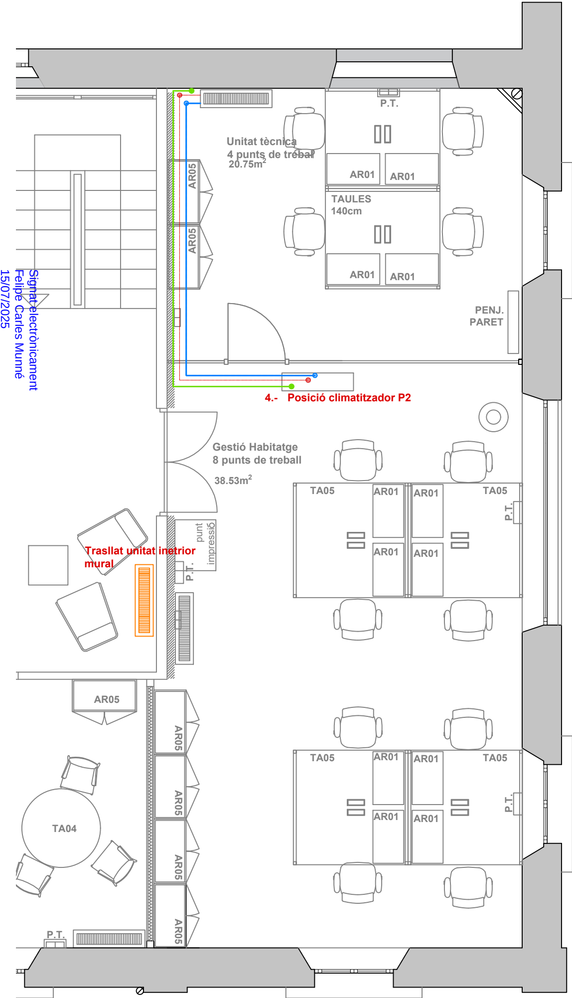
PLANTA PRIMERA
