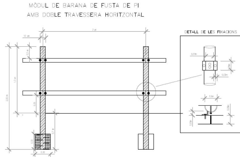
Figura 11. Disseny de la tanca de fusta amb doble travessera horitzontal.
