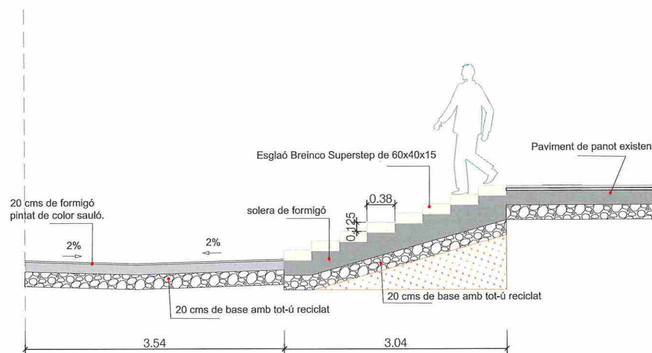
SECCIÓ E-E' PLAÇA NORD SECCIÓ ESCALA
