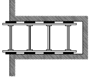
Rases amb apuntalament per sobrecàrrega
