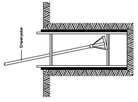
Rases amb apuntalament per sobrecàrrega
