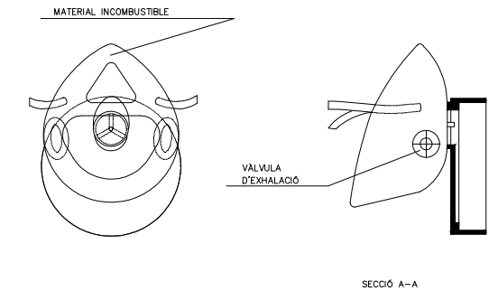
MÀSCARA ANTIPOLS
