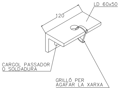
DETALL B
