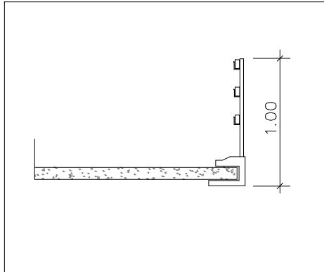
DETALL DE COL.LOCACIÓ DE LES BARANES DE LA VORA DE LA LLOSA
