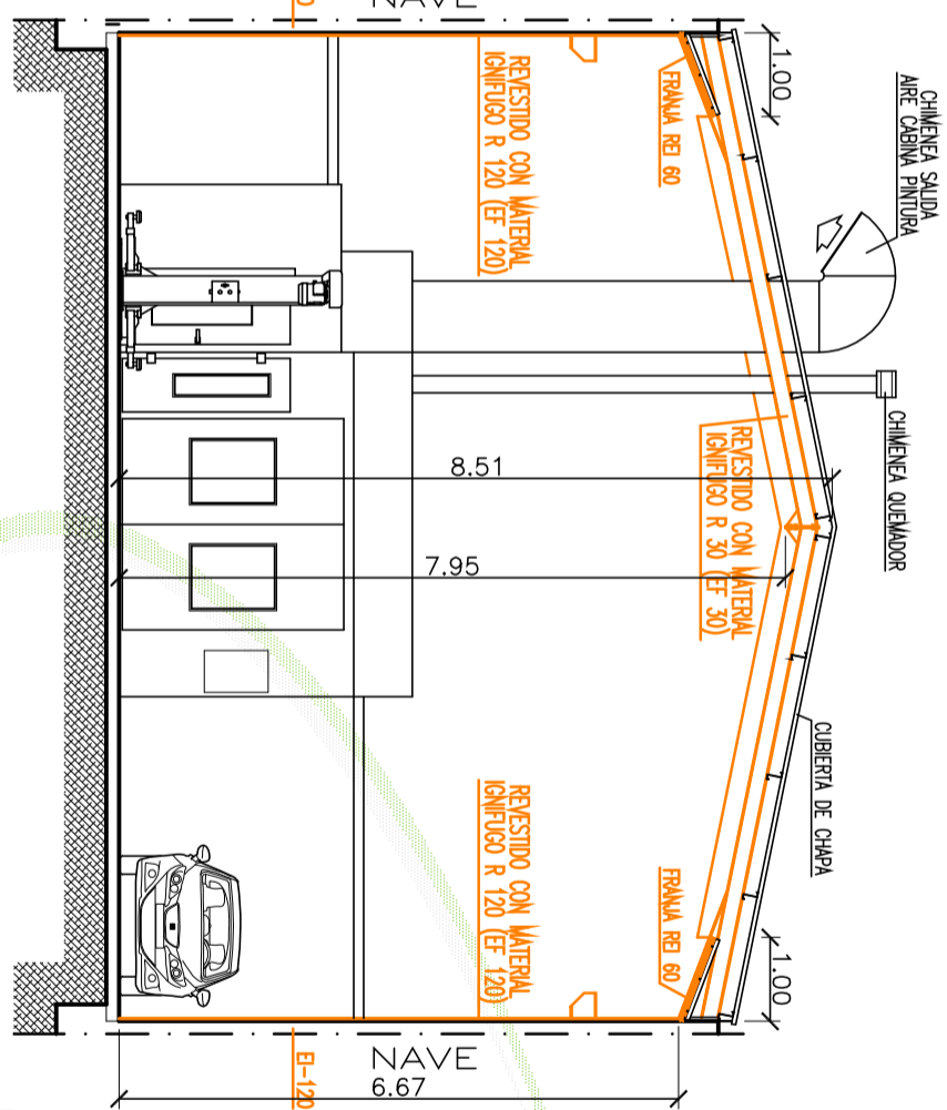
SECCIÓN C-D
