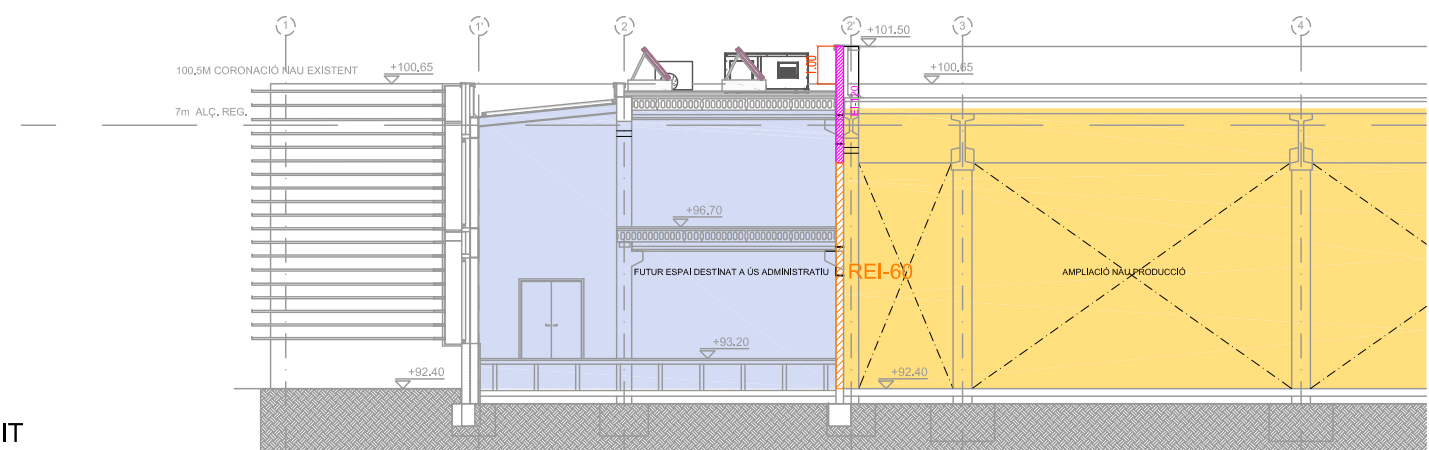
SECCIÓ LONGITUDINAL AMPLIACIÓ NAU PRODUCCIÓ ESCALA 1/100
