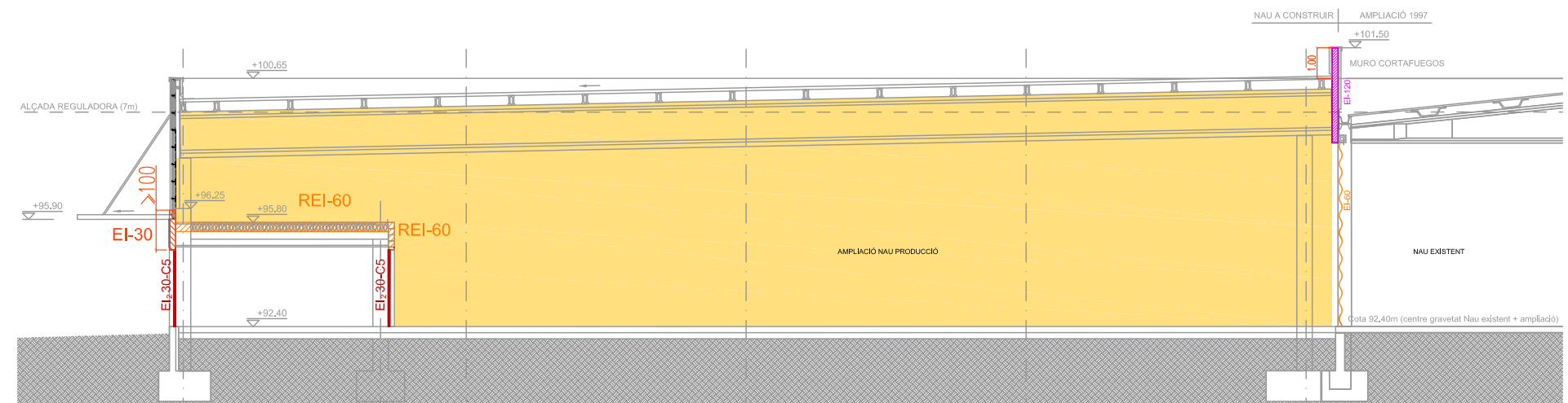
SECCIÓ TRANSVERSAL AMPLIACIÓ NAU PRODUCCIÓ ESCALA 1/100
