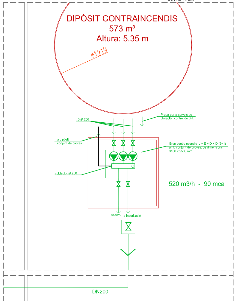
DIPÒSIT I SALA DE BOMBES AMPLIACIÓ NAU PRODUCCIÓ ESCALA 1/100
