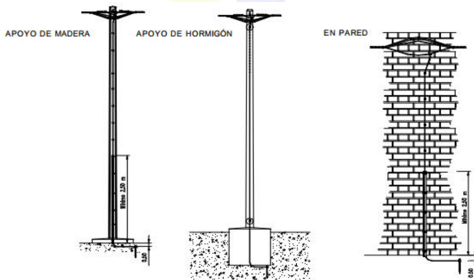
Figura 1. Posada a terra del neutre
