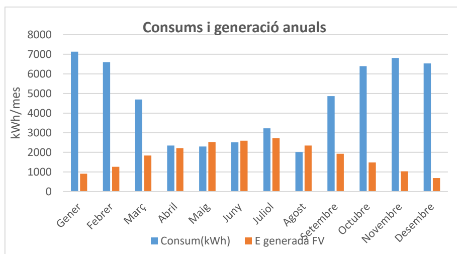
Figura 9 Producció d'energia fotovoltaica i consums mensuals.
