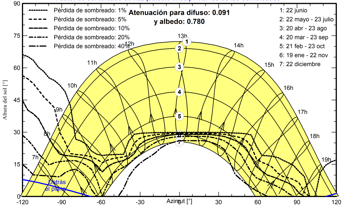
Factor de sombreado de haz (cálculo lineal) : Curvas de iso-sombreados
