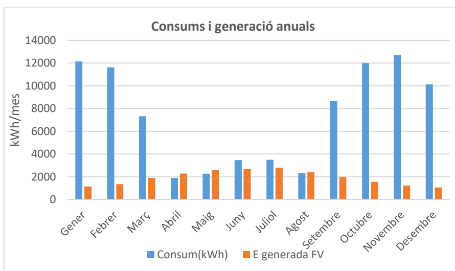
Figura 9 Producció d'energia fotovoltaica i consums mensuals.
