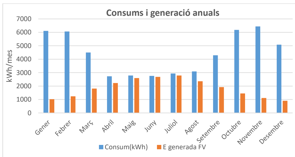
Figura 9 Producció d'energia fotovoltaica i consums mensuals.
