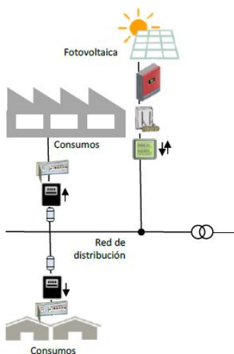
Figura 7 Mode de connexió a través de xarxa amb autoconsum col·lectiu. Font: IDAE
