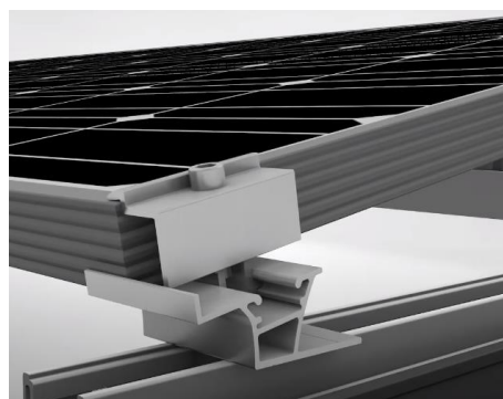
Pletinas I "pinses" de subjecció
